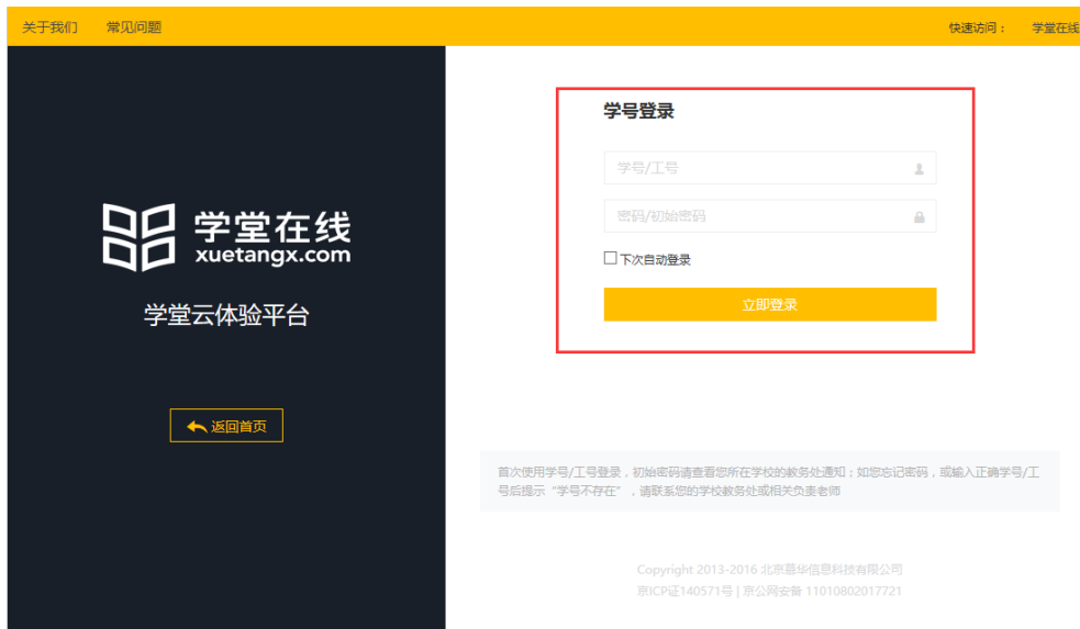
图 3：登录页面
